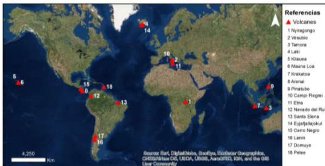
Figura 1: Localización de los volcanes mencionados en el presente trabajo.
